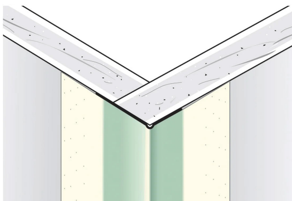
Illustration af hjørneprofilens placering på et udvendigt hjørne.
